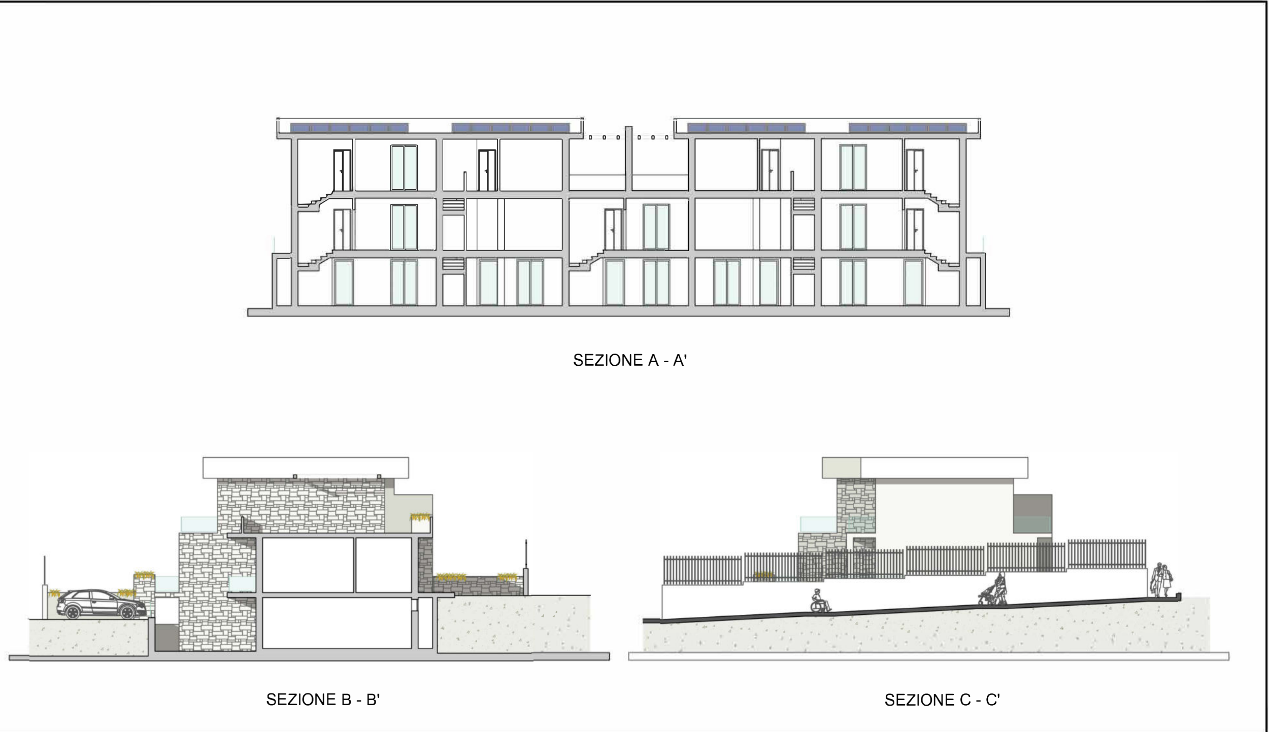
Sezione longitudinale, trasversale e sulla rampa - Scala 1:200
