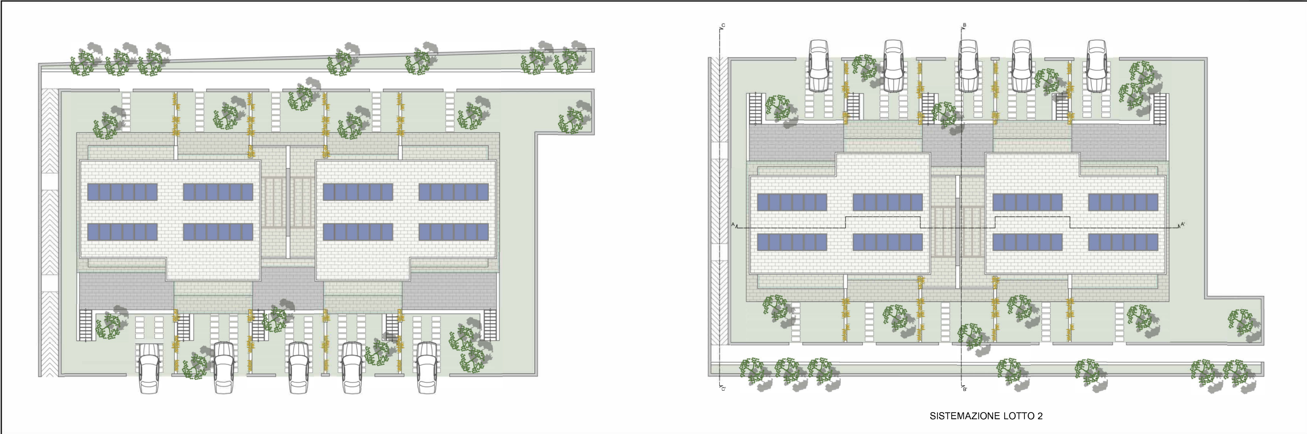
Piante e prospetti - Scala 1:200
